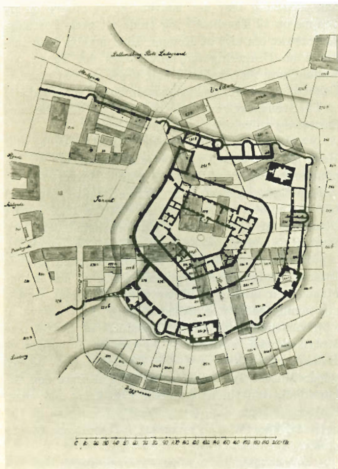
Fig. 2. Kalundborg Slots Grundplan, sammenarbejdet med Matrikelkortet af Landinspektør A. M. Rørup.
